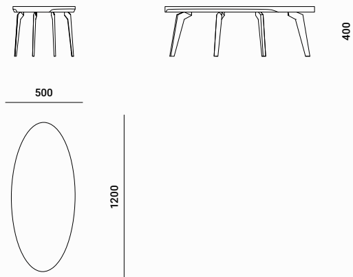
Jolie - Coffee Table Code : CT 120R
