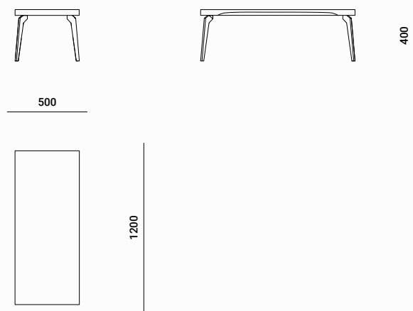
Jolie - Coffee Table Code : CT 120R
