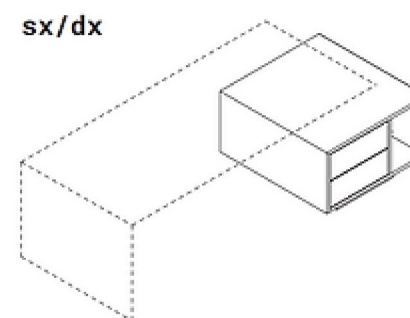
L 90 P 98 H 59,2
