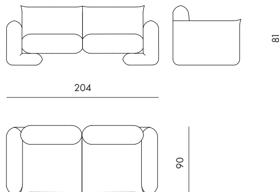
Era : 2 Seater Code : 2S
