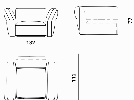
Oasi : Armchair Code : AR
