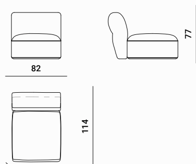
Oasi : Central element Code : CM
