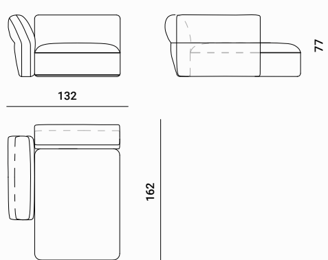
Oasi : Chaise lounge maxi with left armrest Code : CLML
