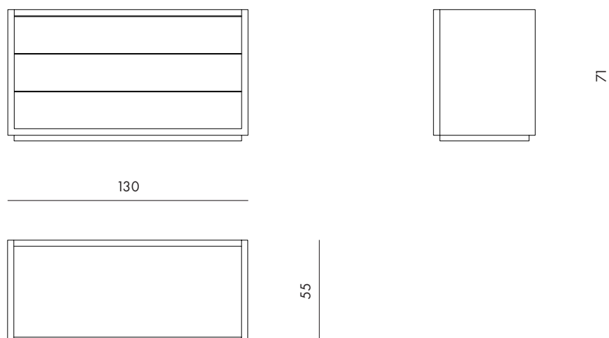
Jacob - Commode Code : COM130
