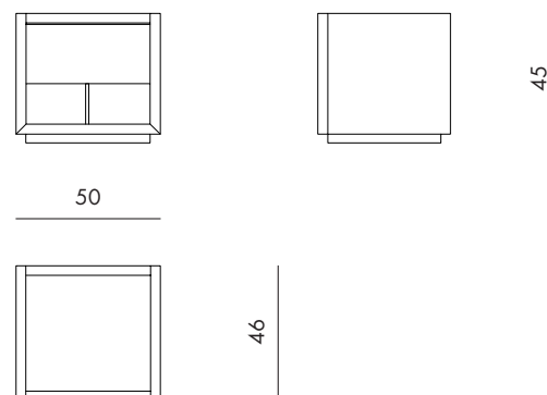
Jacob - Night Stand Code : NST50
