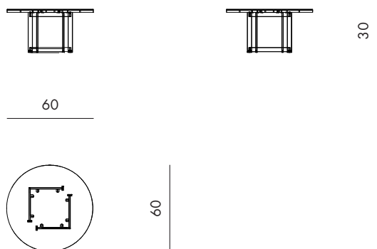
Puzzle - Service Table Code : STL 60RO
